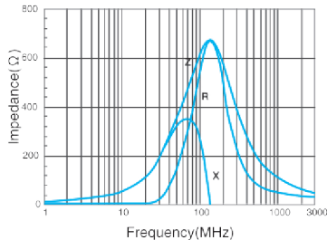
SKCB2012-601
