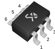
SOT-363
