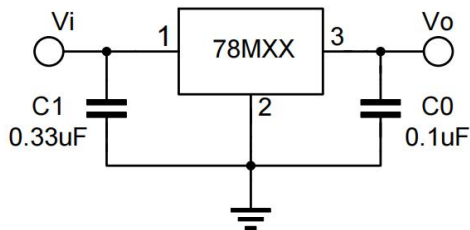
Fig.1 DC PARAMETERS
